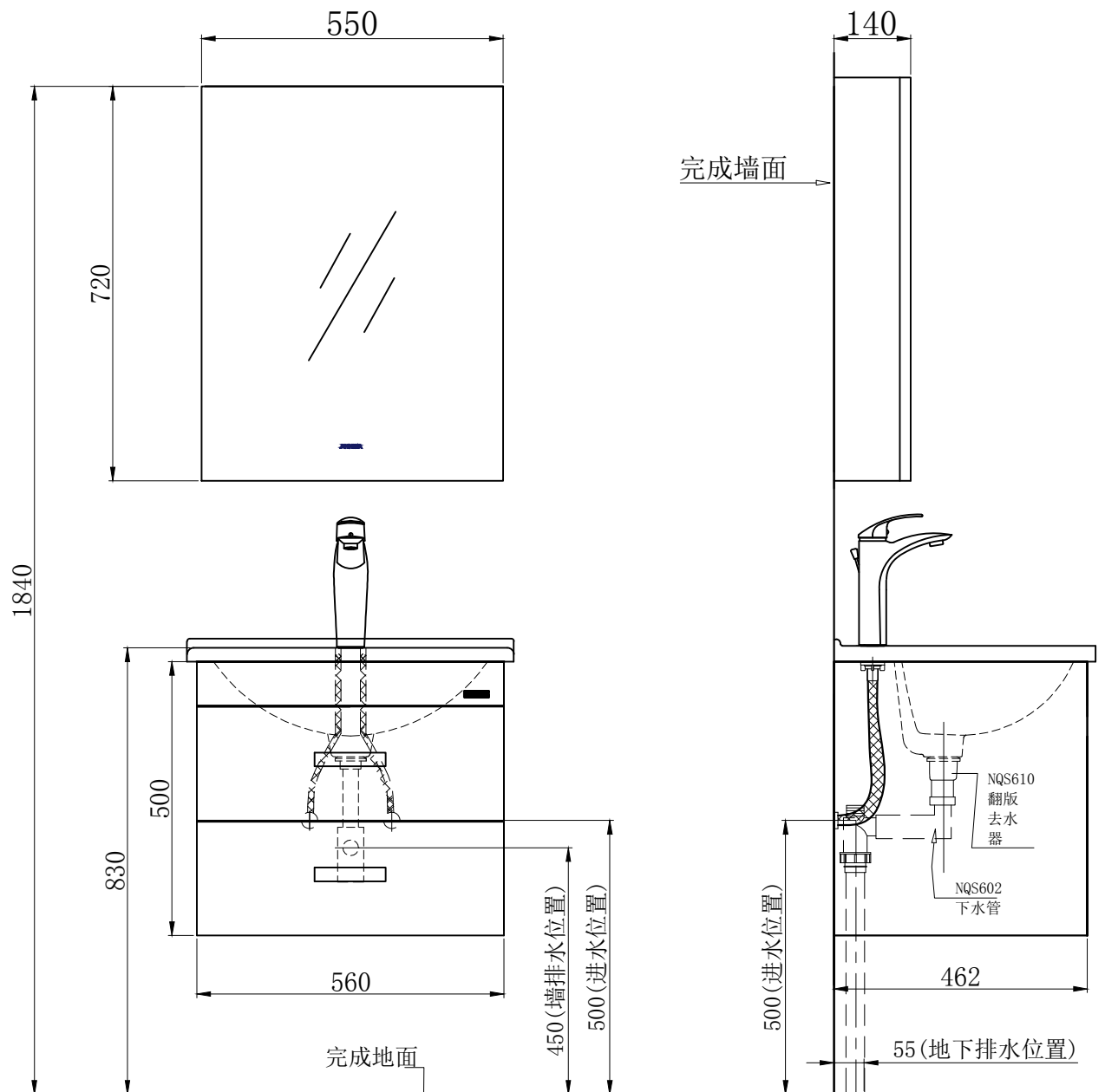
N3D60G10-L 水电安装图 (建议安装尺寸)
