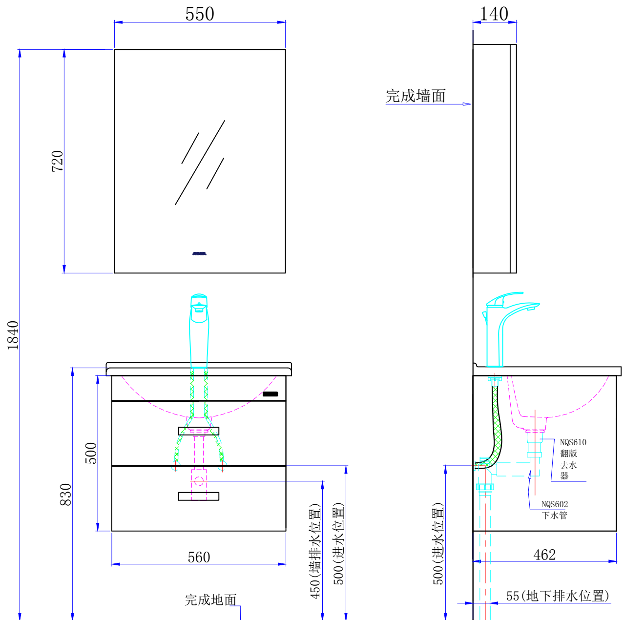
N1D60G10-L 水电安装图 (建议安装尺寸)
